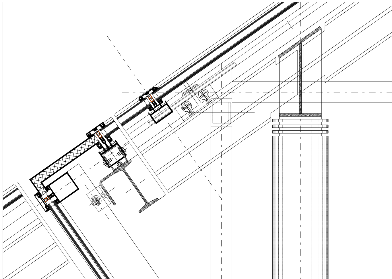
ÜVEGTETŐ RÉSZLETRAJZ M=1:2
