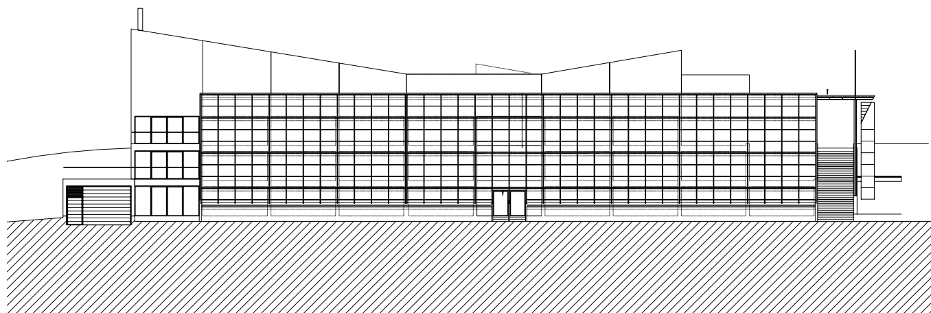
KELETI HOMLOKZAT M=1:400
